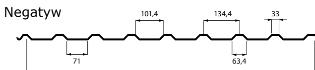
Szerokość efektywna 1075
