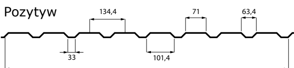
Szerokość efektywna 1075
